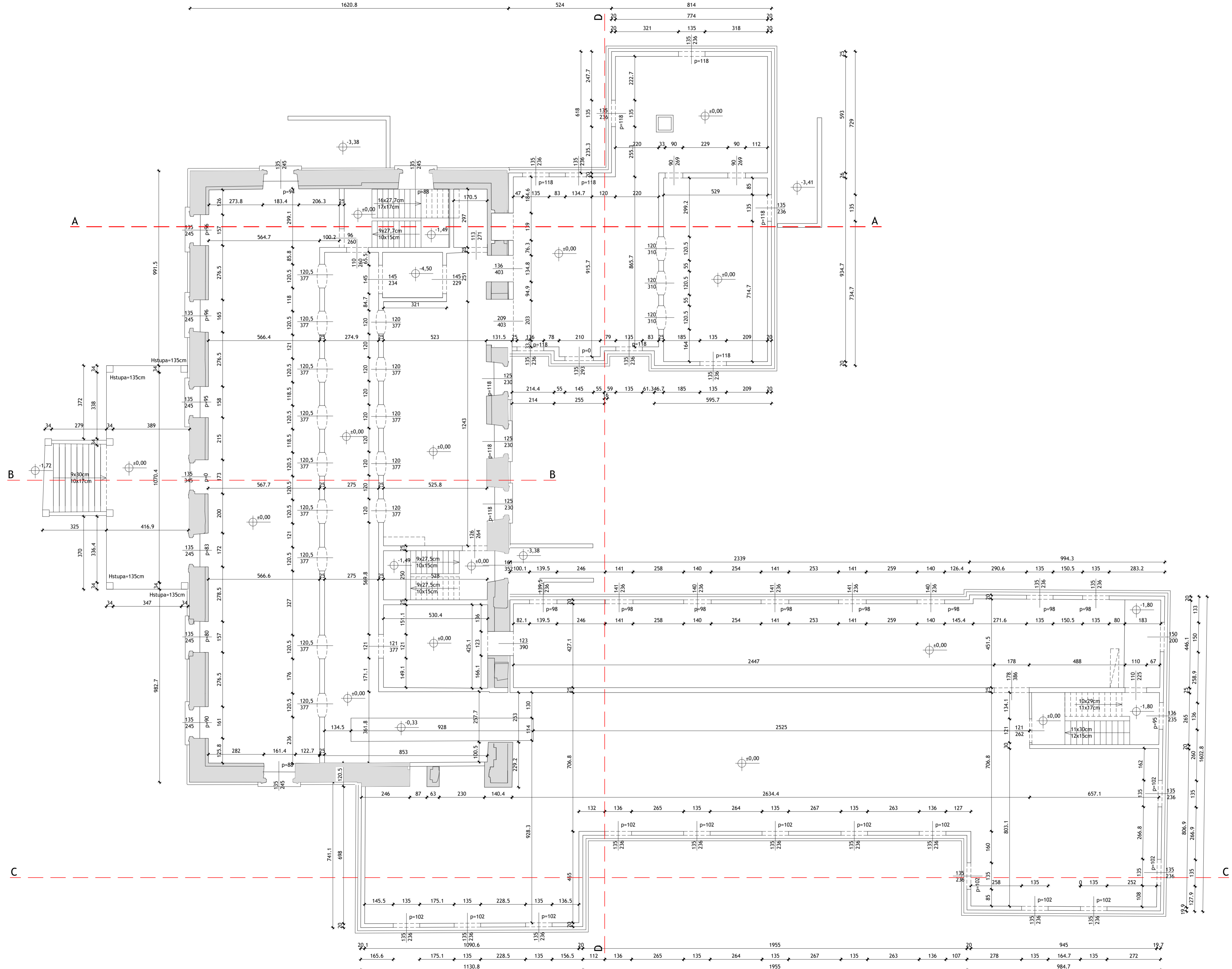
TLOCRT PODRUMA - snimak izvedenog stanja - mj 1:100
