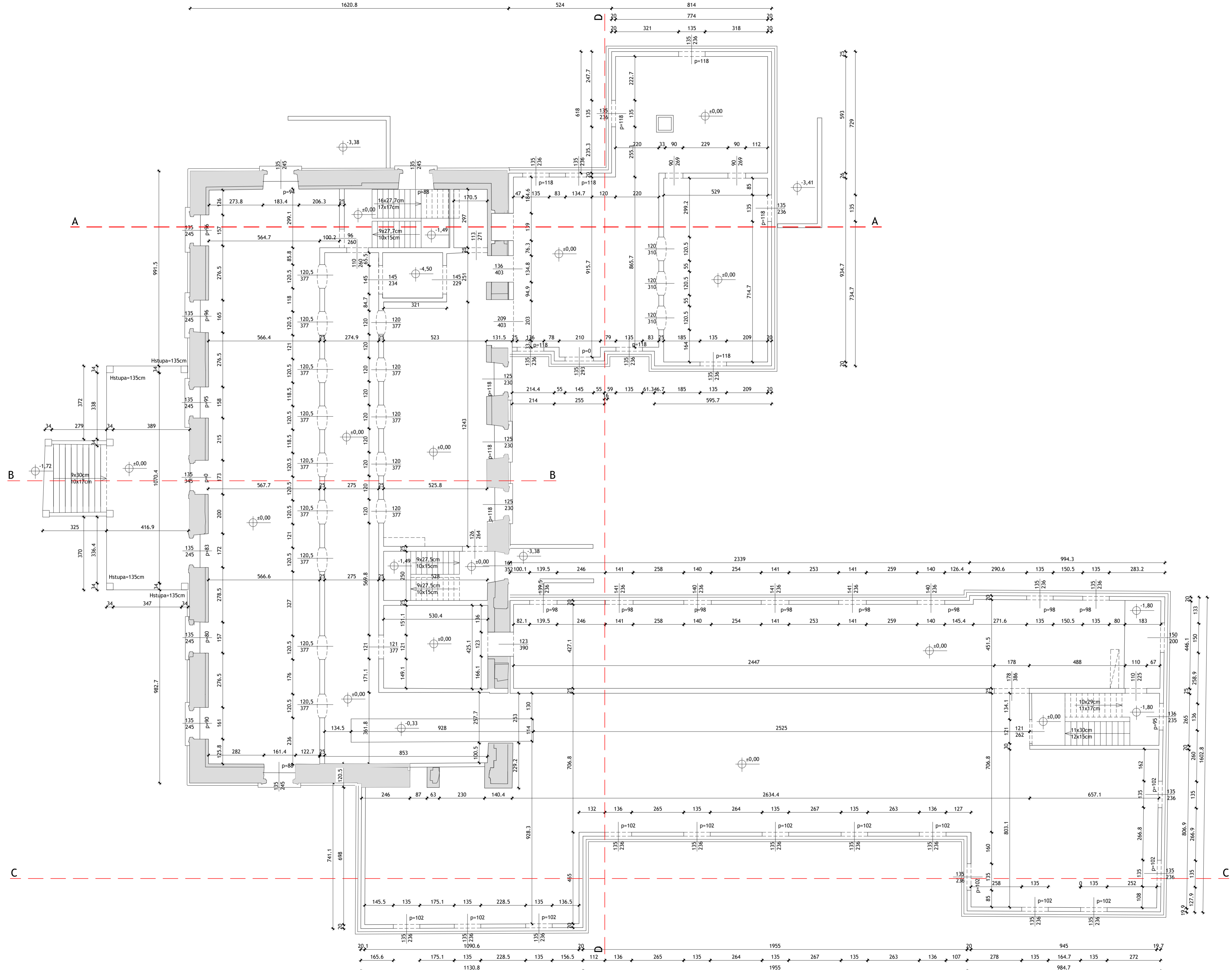
TLOCRT PRIZEMLJA - snimak izvedenog stanja - mj 1:100
